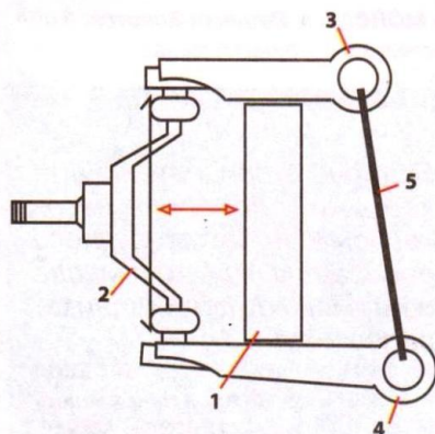
Рис. 1 Сборка суппорта 1 — опора d 57x260 мм, 2 — кулак, 3 и 4 — верхний и нижний рычаги, 5 — оттягивающая проволока
