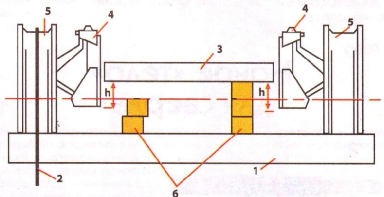
Рис. 3 Сборка моста 1 — швеллер № 18 (180 мм), 2 — стягивающая проволока, 3 — балка d 76 мм, 4 — суппорты, 5 — диски, 6 — бруски 10x10x200 см
